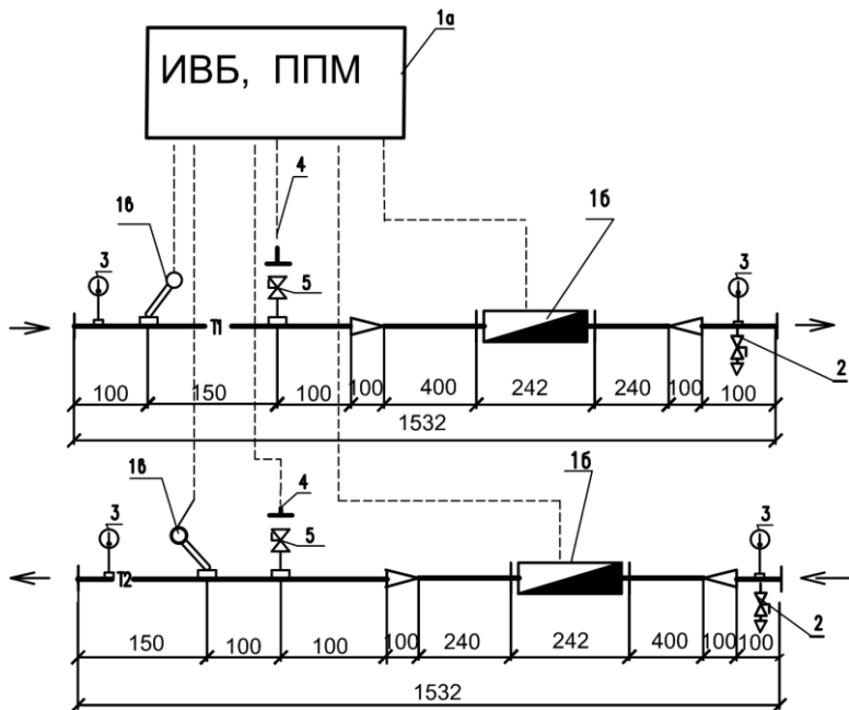
Рис.8 Принципиальная схема УУМ-125-80
