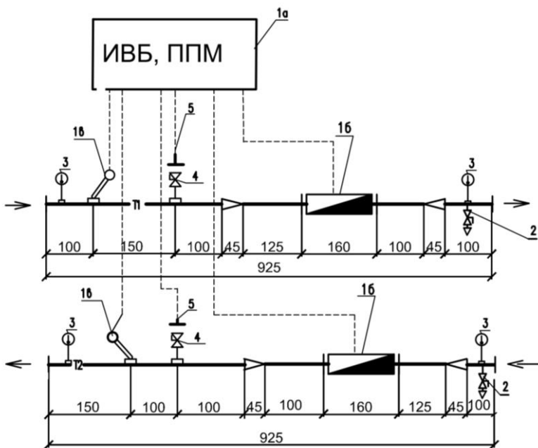
Рис.2 Принципиальная схема УУМ-50-25
