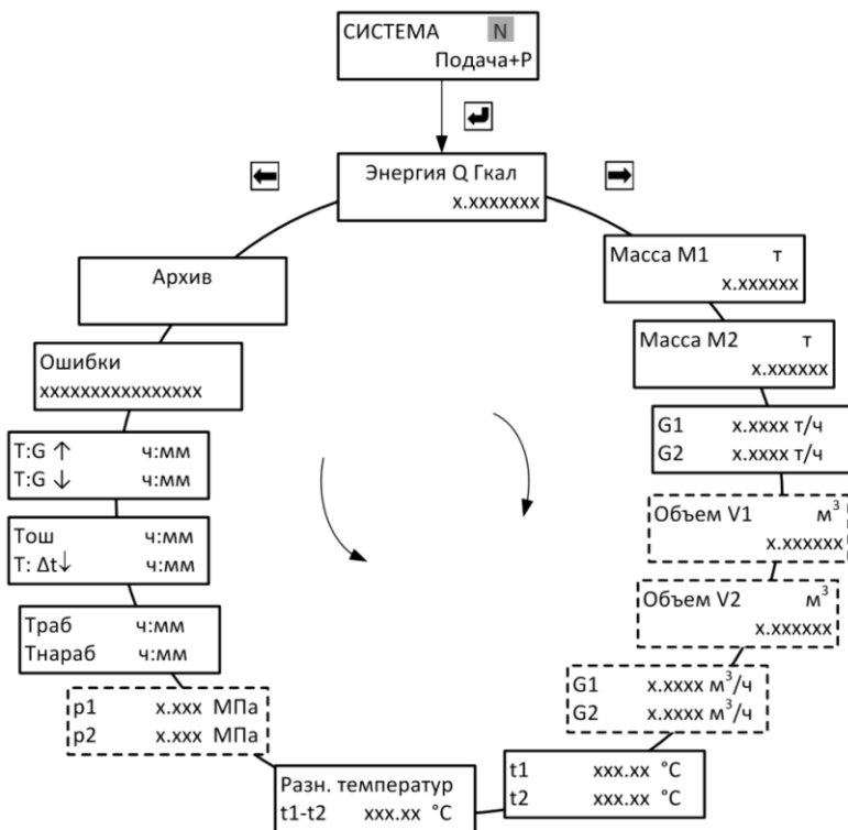
Рис. 14 Режим «рабочий» для схемы «Подача_P»
