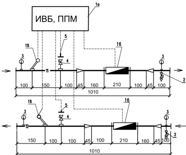
Рис.3 Принципиальная схема УУМ-50-32
