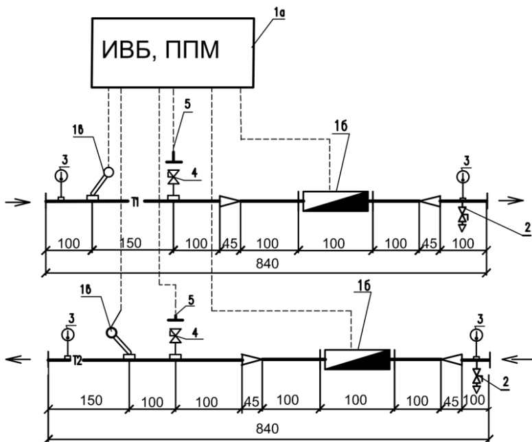
Рис.1 Принципиальная схема УУМ-50-15
