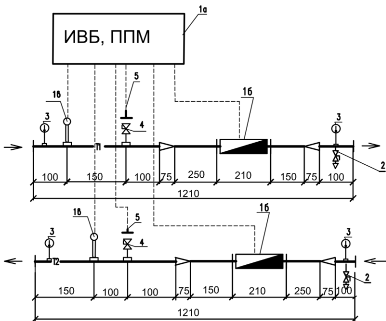
Рис.5 Принципиальная схема УУМ-80-50
