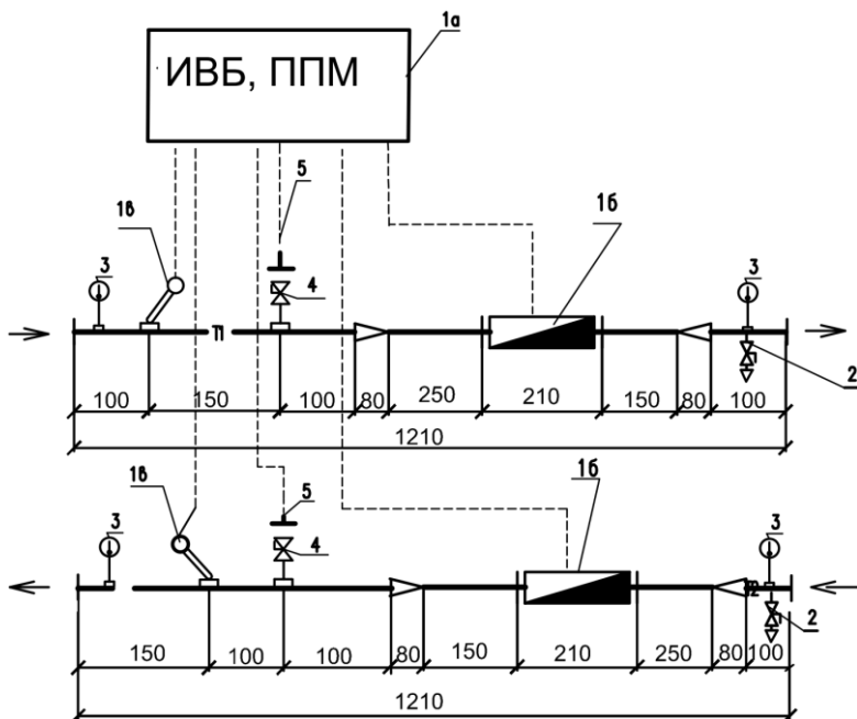
Рис.6 Принципиальная схема УУМ-100-50
