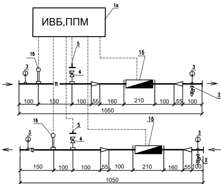
Рис.4 Принципиальная схема УУМ-65-32
