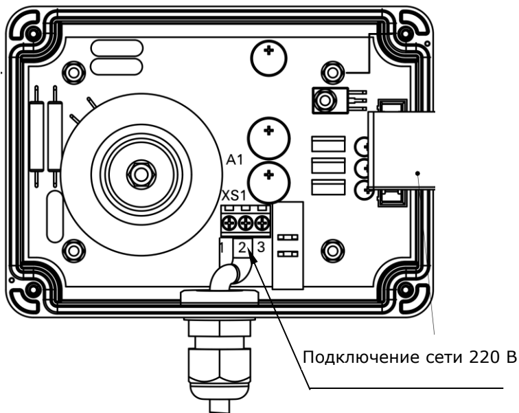
Рис 10 Схема подключения УУМ к сети 220 В переменного тока при комплектации ППМ (ТСМ, РСМ-05.05, РСМ-05.07)
