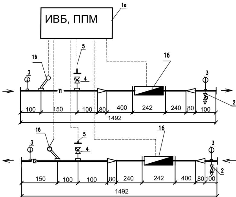
Рис.7 Принципиальная схема УУМ-100-80 (80-80)
